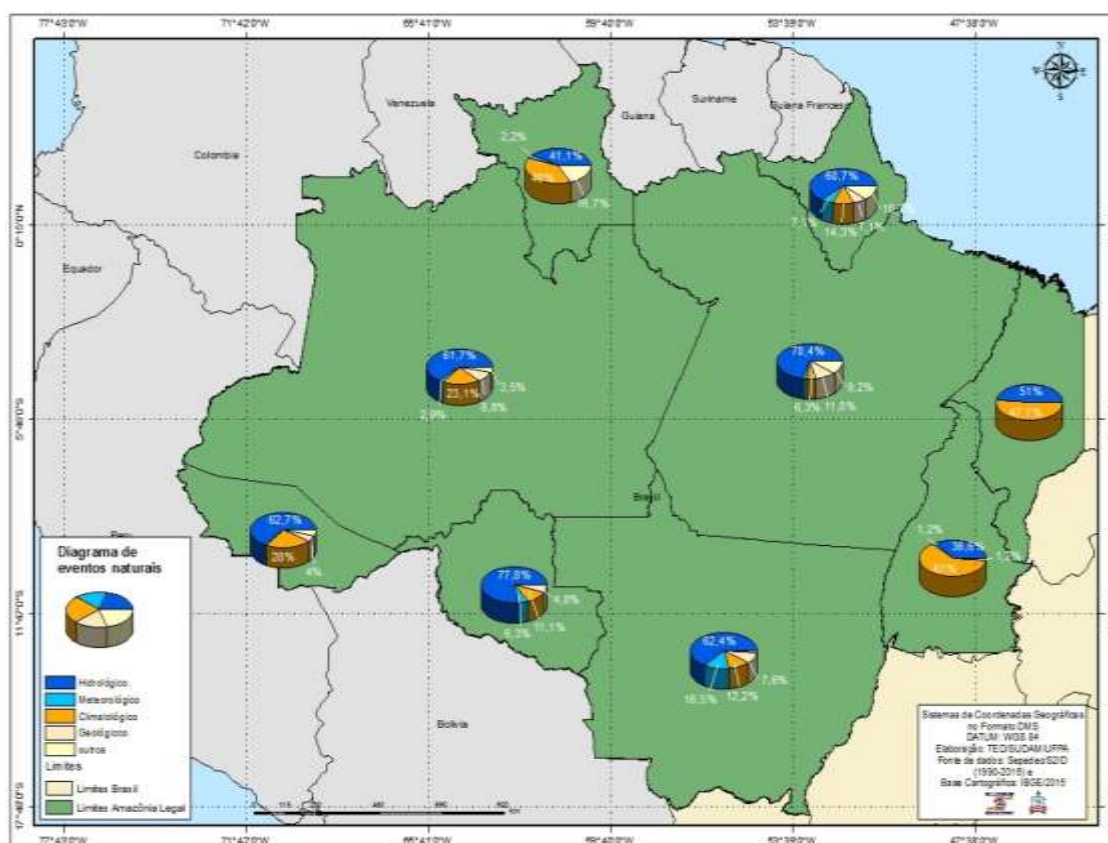
Figura 7 - Representação percentual das ocorrências de desastres naturais na Amazônia legal.
