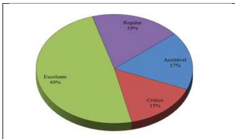
Figura 30 - Categorização de erros avaliativos resultantes das previsões emitidas no período de 2016-2018 para o município de Boa Vista.
