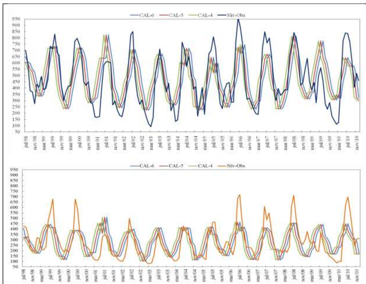
Figura 26 - Comportamento do tempo de resposta das componentes climáticas na variação fluviométrica de níveis máximos no intervalo de 1998-2010.
